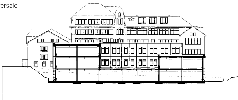
Coupe longitudinale
